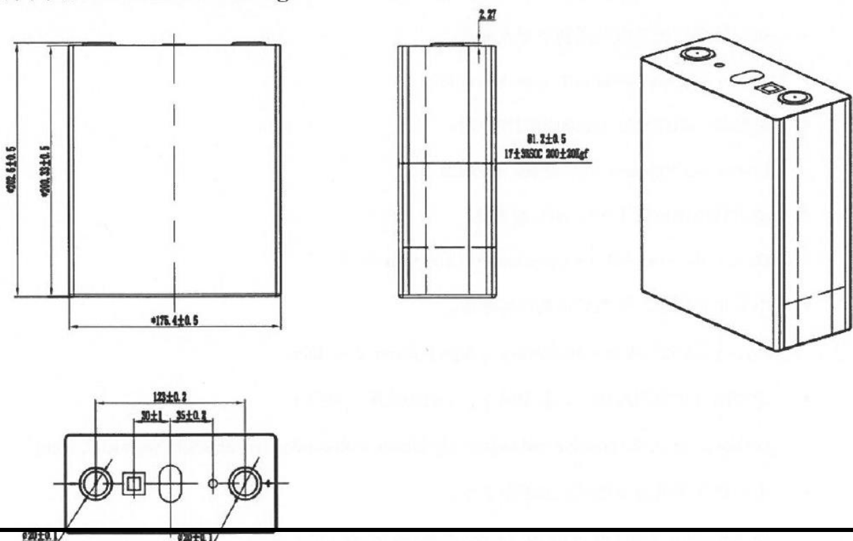
电芯尺寸 Cell Dimension
